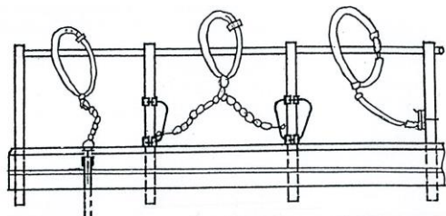
Attache télescopique (tampou dans le sol)
